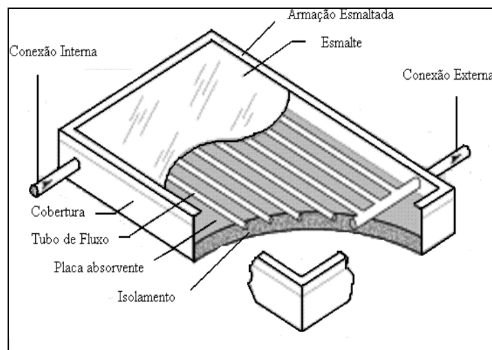
Figura 1: Placa Coletora para fins fotovoltaicos
