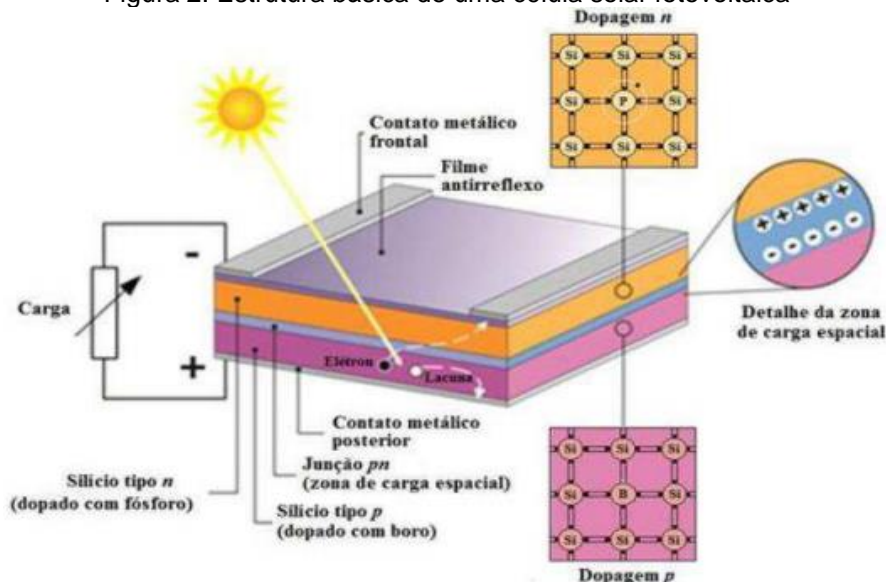
Figura 2: Estrutura básica de uma célula solar fotovoltaica
